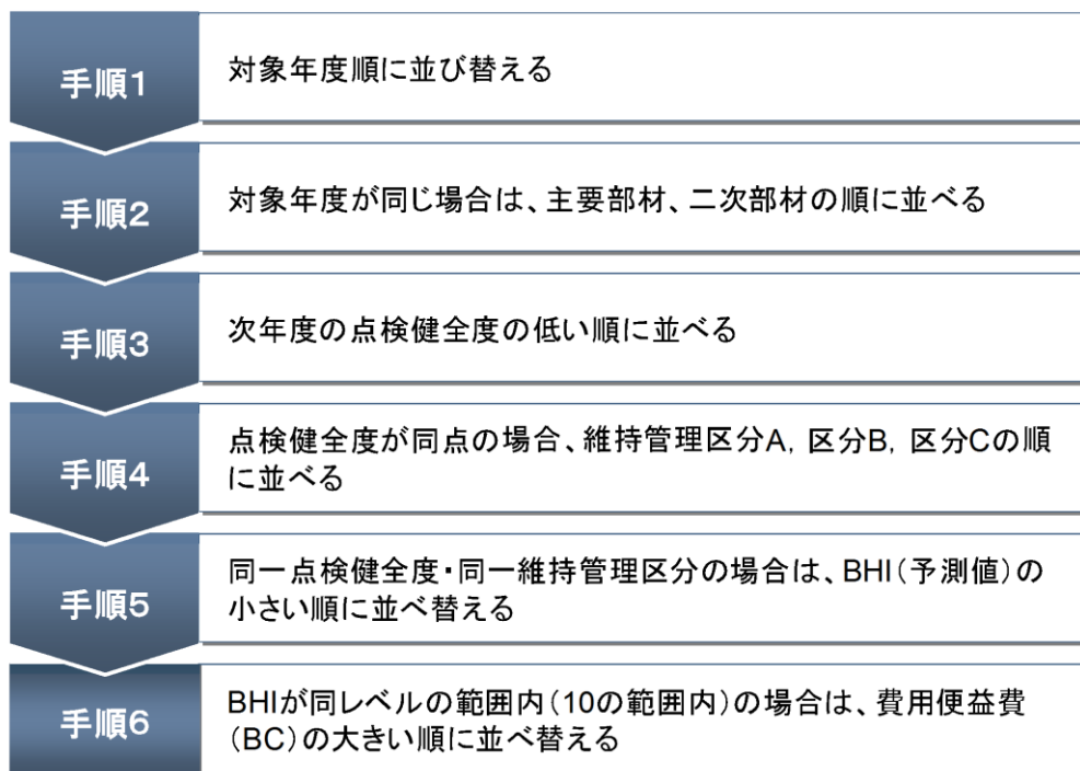
図 3.6 補修補強の優先順位付け手順
