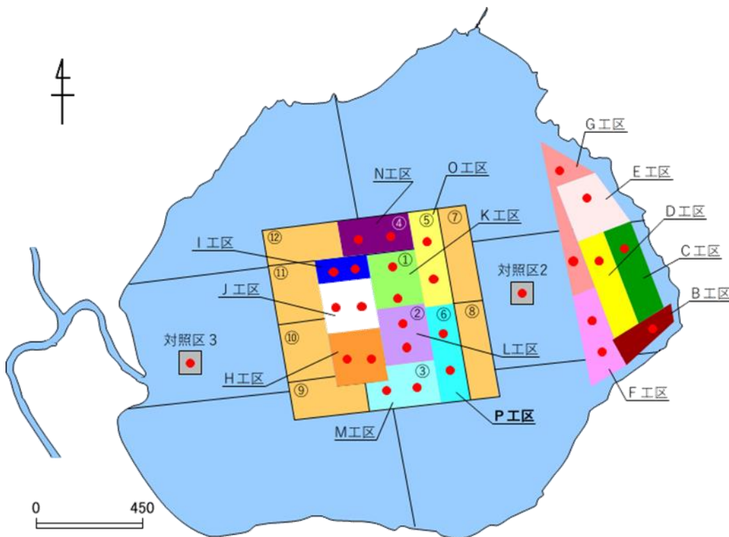
覆砂区域位置図 (R6 実施:P 工区) (参考:R5 実施:O 工区)
