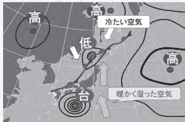
▲大雨になりやすい気圧配置
