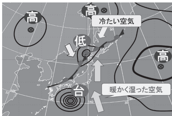
▲大雨になりやすい気圧配置
