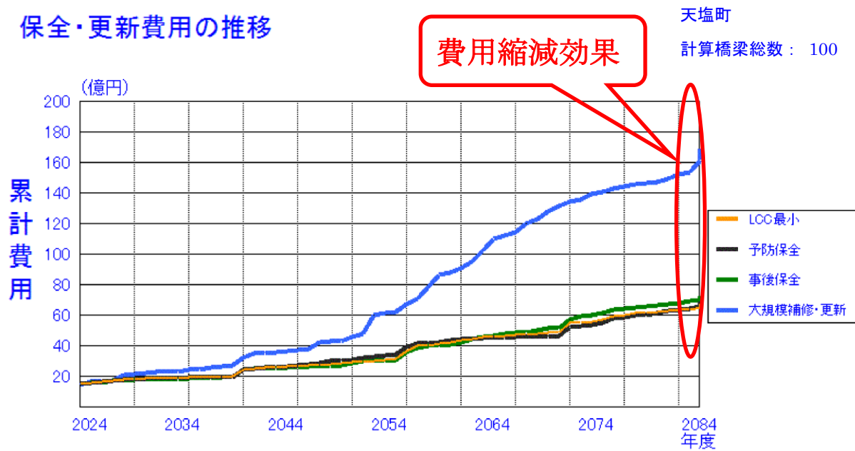
図-5 保全・更新費用の推移（累計費用）
