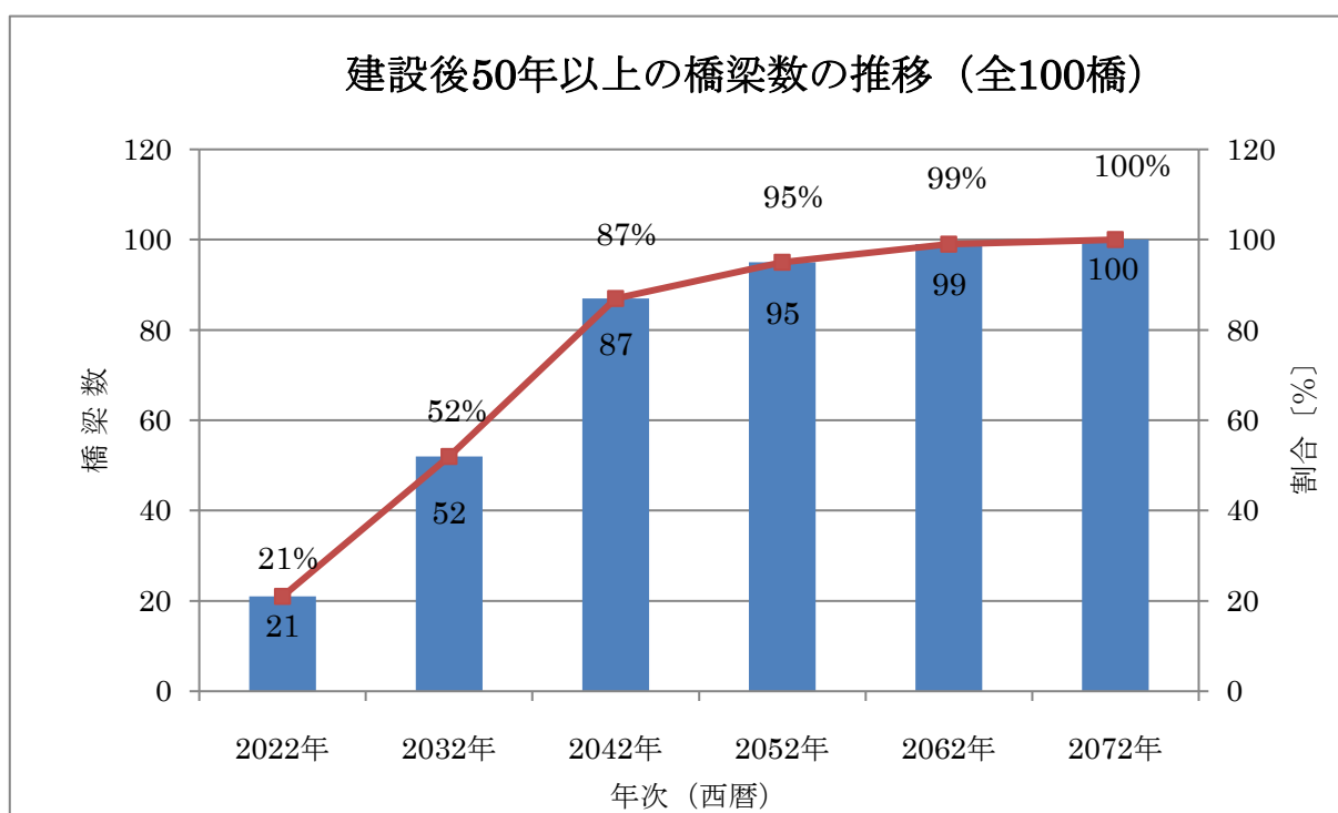
図-1 天塩町における建設後 50 年以上の橋梁数の推移
