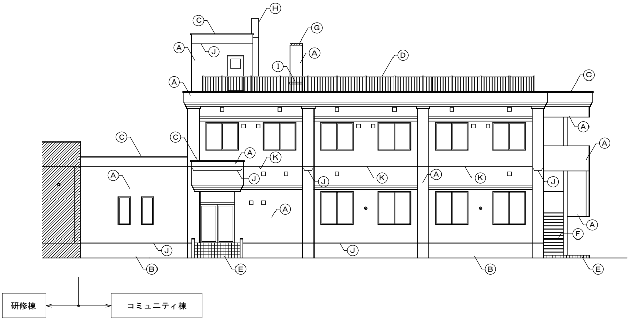
東面立面図
