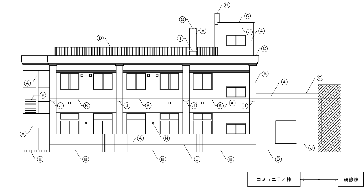
西面立面図
